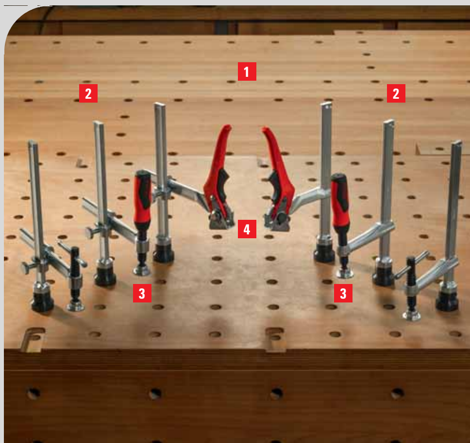
Adattatore per banchi da lavoro TW16AW
