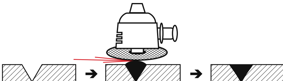
Perfetta spianatura delle saldature con FLEXCELLENCE .
