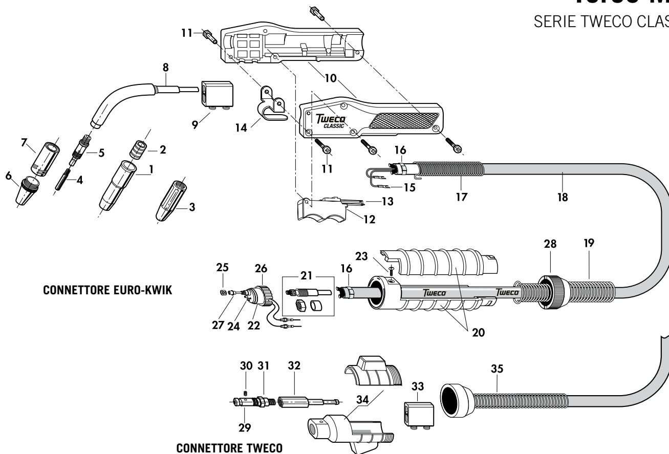
LISTA PARTI DI RICAMBI CLASSIC NO.2
