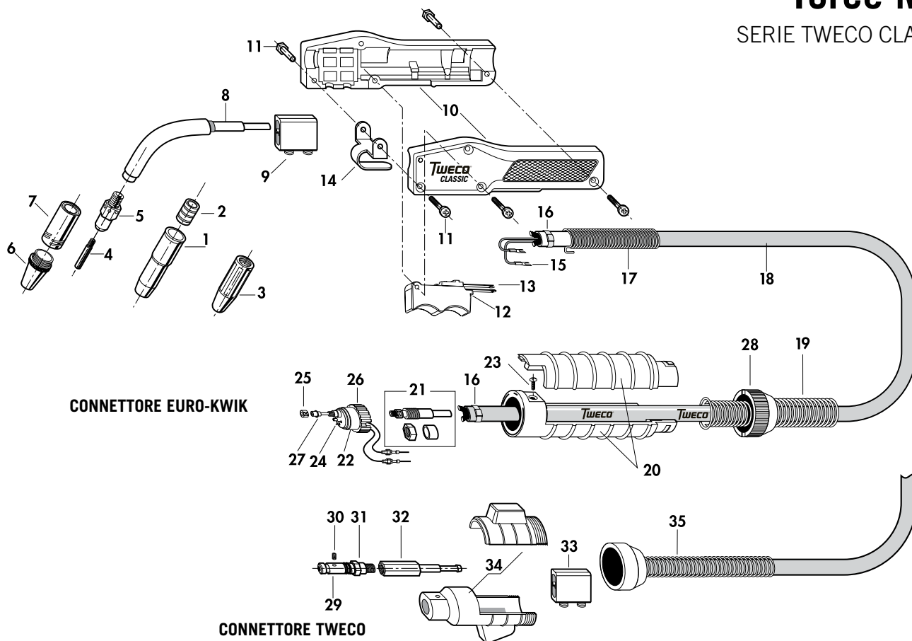
LISTA PARTI DI RICAMBI CLASSIC NO.3
