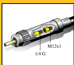
Torcia con connessione MK
