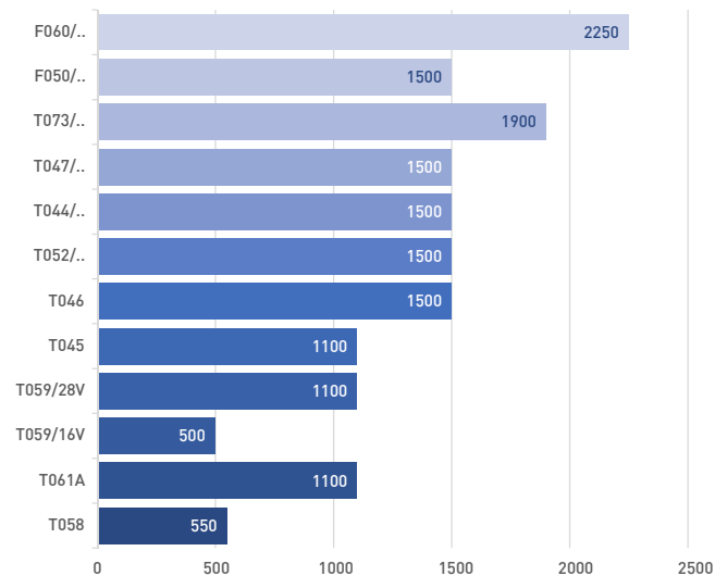
Potenza (W)
