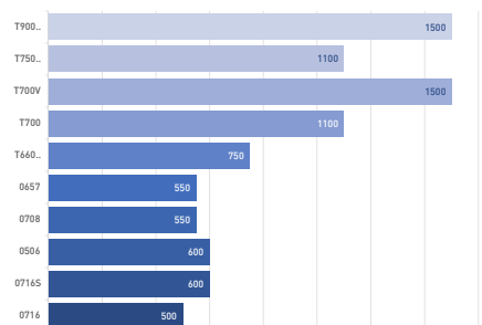
Potenza (W)
